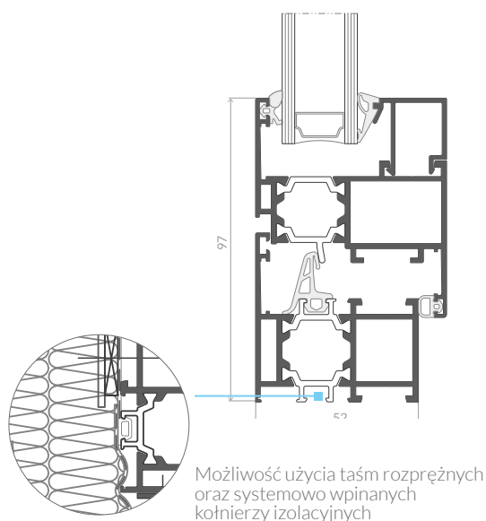
Przekrój okna otwieranego
