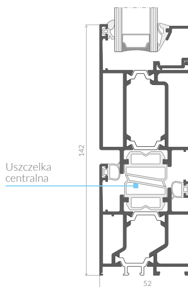
Przekrój drzwi otwieranych do wewnątrz
