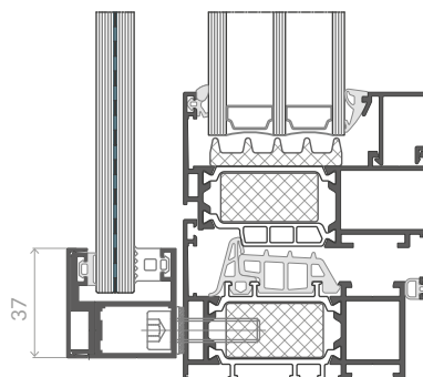
Mocowanie balustrady do okna otwieranego
