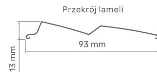
Przekrój lameli
